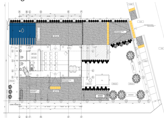
IMAGEN 39 PLANTA PROPUESTA DE ARQUITECTURA SEDE SOCIAL
