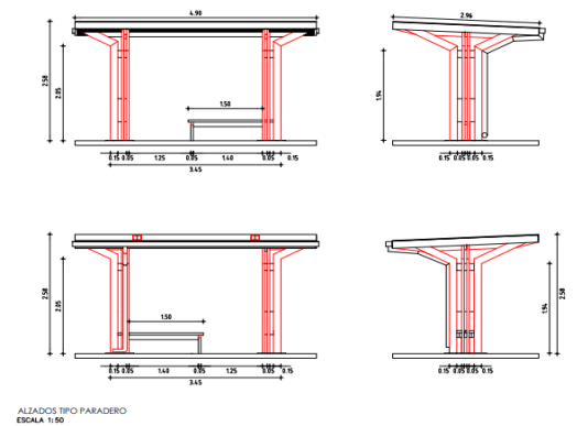
IMAGEN 43 PLANIMETRIA DEL DISEÑO DE PARADEROS URBANOS
