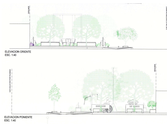
IMAGEN 42 PLANIMETRÍA PROYECTO "MEJORAMIENTO DE VEREDAS URBANAS Y ESPACIO PÚBLICO SECTOR SUR PONIENTE"
